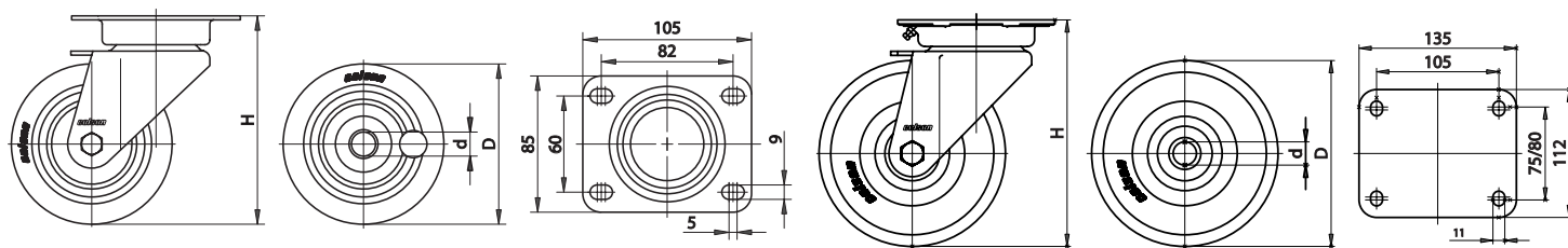
Afmetingen voor wieldiameter 70 tot 125 mm
